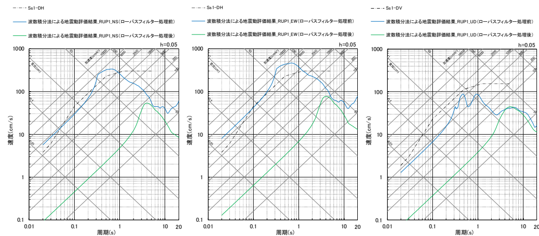
A-17断層_基本震源モデル_RUP1 グラフ
